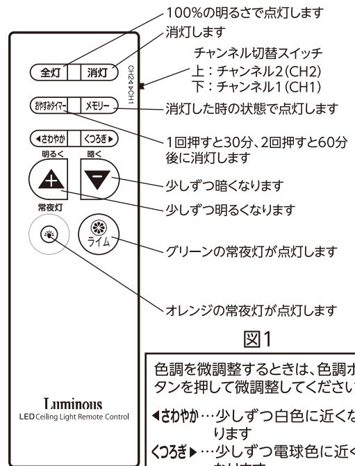
リモコン 図1
